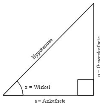
Bild 41. Ein rechtwinkliges Dreieck hat einen 90-Grad-Winkel.
