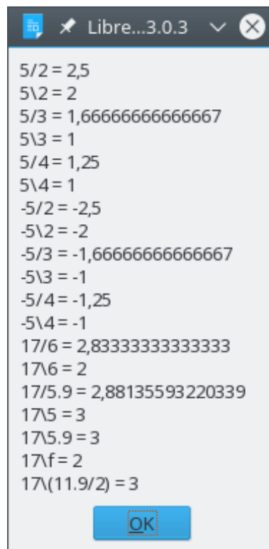
Bild 30. Ganzzahlige Division.
